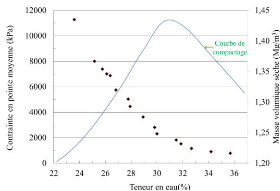
Figure 6. Contrainte en pointe moyenne à 20^\circ\text{C} à différentes teneurs en eau et masses volumiques sèches pour l'illite.
