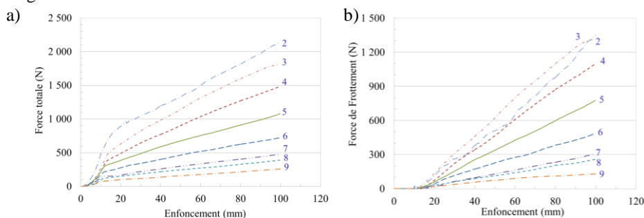
Figure 7. a) Force totale ( Q_t ); b) Force de frottement ( Q_f - Q_p ) en fonction de la profondeur pour les éprouvettes d'illite.
