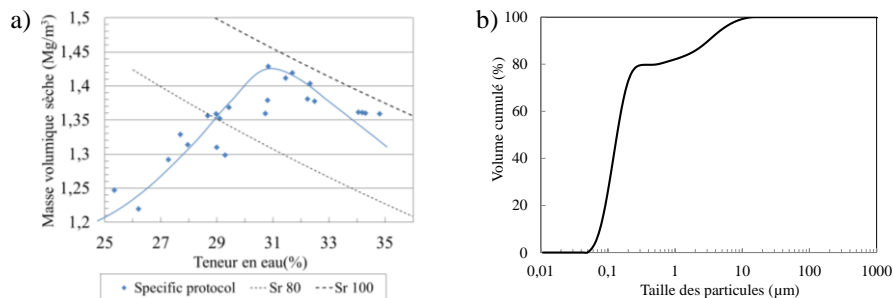
Figure 2. a) La courbe de compactage ; b) Distribution de la taille des particules
