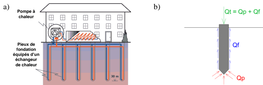
Figure 1. a) Schéma de fonctionnement de pieux énergétiques [LAP 10] ; b) Force portante d'un pieu.
