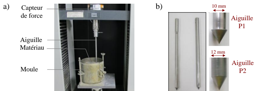
Figure 3. a) Dispositif expérimental de l'essai pénétrométrique à l'aiguille ; b) Deux différentes aiguilles P1 et P2.
