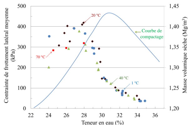
Figure 10. Contrainte de frottement latéral moyenne à 1, 20, 40 et 70°C à différentes teneurs en eau et masses volumiques sèches pour l'illite
