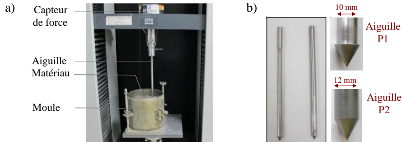
Figure 3. a) Dispositif expérimental de l'essai pénétrométrique à l'aiguille ; b) Deux différentes aiguilles P1 et P2.
