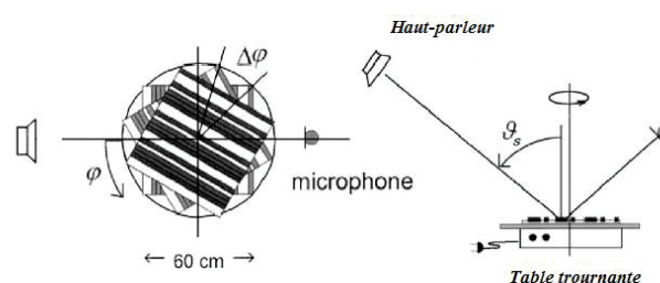
Figure 1 : Principe de la méthode de détermination du coefficient de diffusion en champ libre [1]
