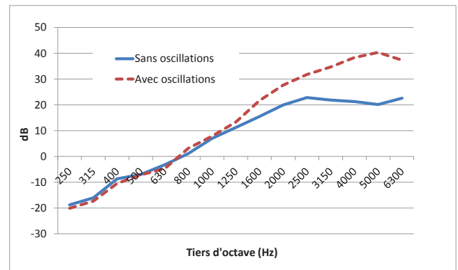
Figure 9 : Spectre des réponses impulsionnelles avec et sans oscillations autour du pic d'impulsion spéculaire réfléchi
