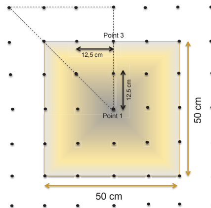
Figure 14 : Points de mesure au-dessus de la cavité
