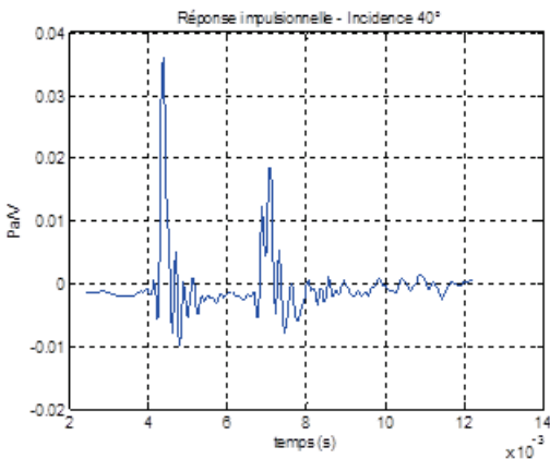
b - Réponse impulsionnelle moyennée sur \varphi (n=10) – Incidence \theta_s = 40^\circ
