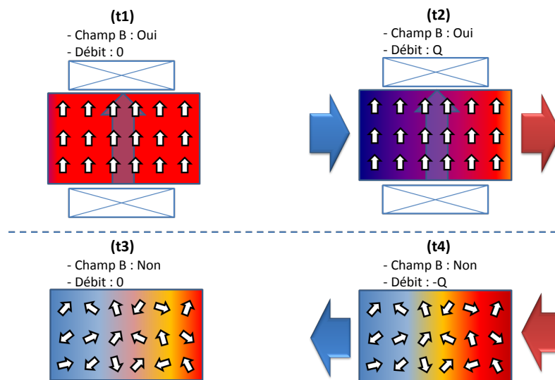
Figure 1 : Principe d'un cycle à régénérateur magnétique actif.
