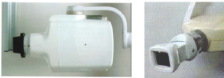
Figures 16 et 17 : Adjonction d'un dispositif collimateur rectangulaire à l'extrémité d'un cône cylindrique (Attal et Kaleka, 2008 ; White et Pharoah, 2014)
