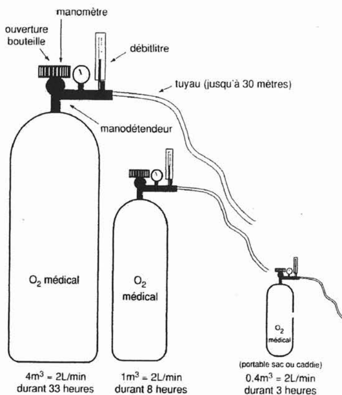
Fig. 2 – Schémas de bouteilles d'oxygène gazeux et de leur détendeur-débitlitre (49)
