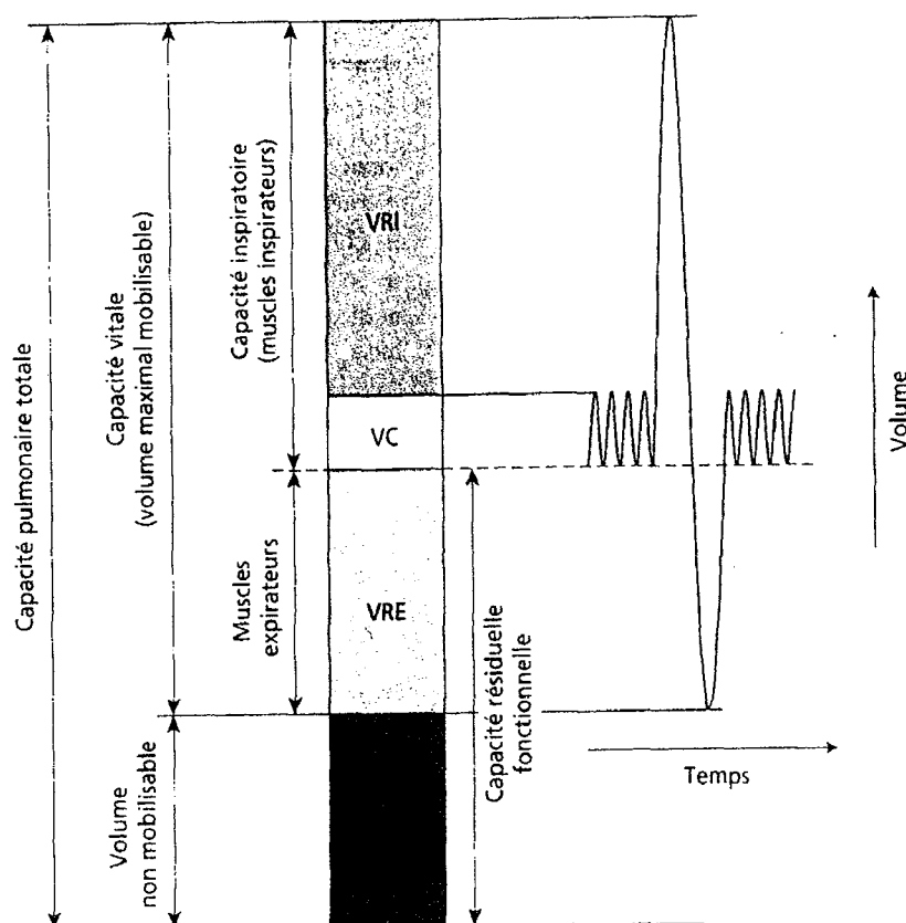
Fig. 13 - Volumes pulmonaires (24)
