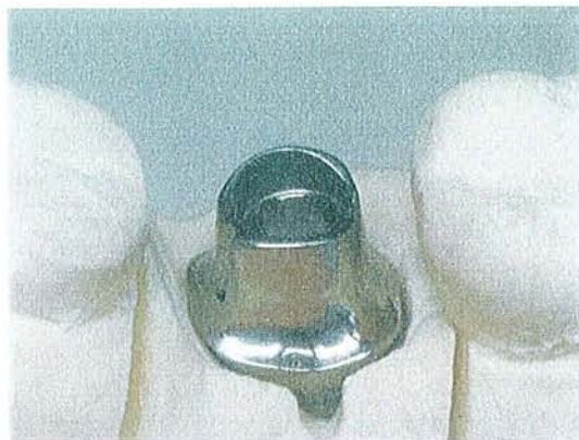
Figure 63 : Pilier Procera sur le modèle de travail.
