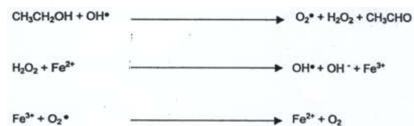
Figure 22 : oxydation de l'éthanol par les radicaux libres (11).
