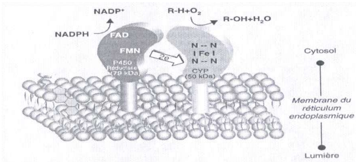
Figure 11 : localisation membranaire et fonction du CYP P450 dans le réticulum endoplasmique (15).
