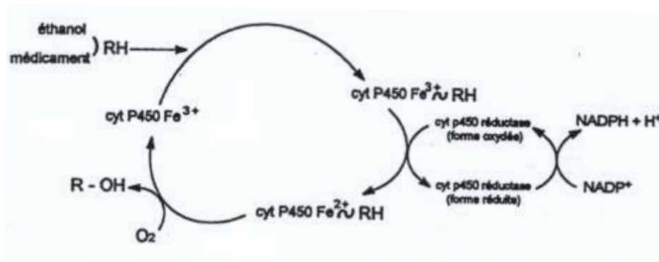
Figure 20 : réaction d'hydroxylation du MEOS (11).
