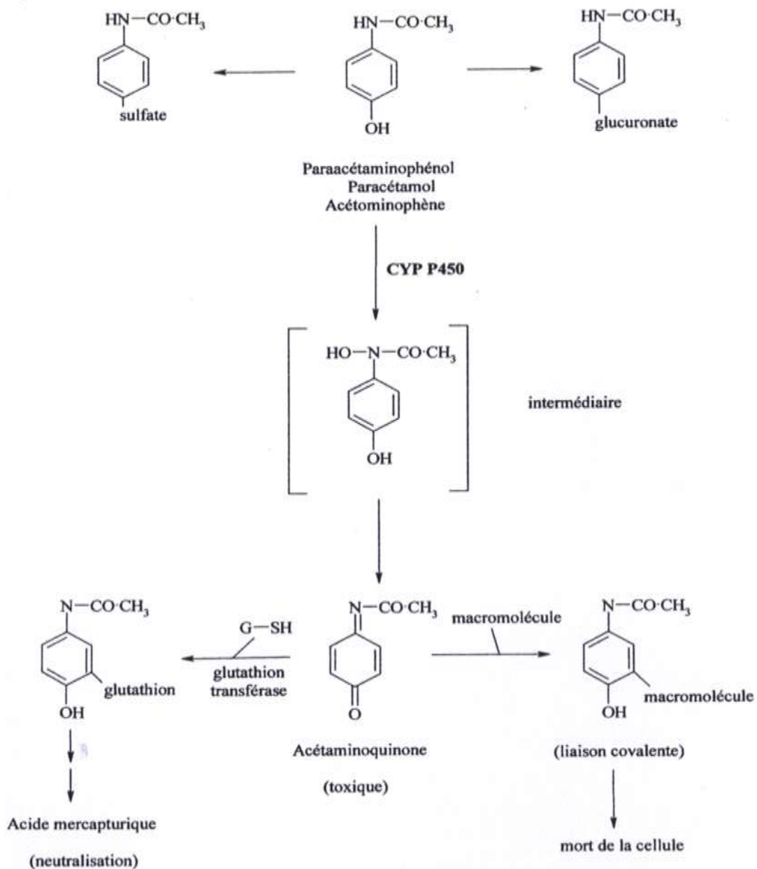
Figure 26 : métabolisme du paracétamol (10).
