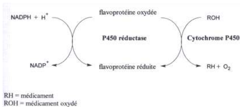
Figure 2 : représentation simplifiée de l'oxydation d'un médicament par le cytochrome P450 (4).
