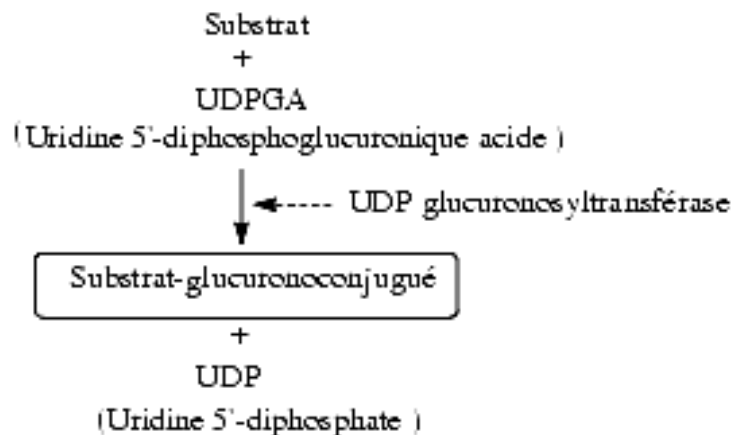
Figure 5 : résumé de la glucuronoconjugaison d'un substrat (2).
