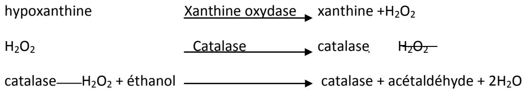
Figure 21 : oxydation de l'éthanol par la voie de la catalase (11).
