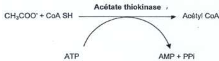
Figure 25 : transformation de l'acétate en acétylCoA.
