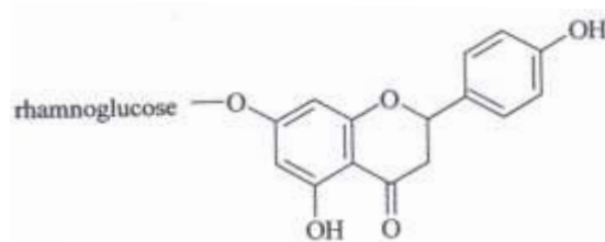
Figure 16 : structure de la naringine (39).
