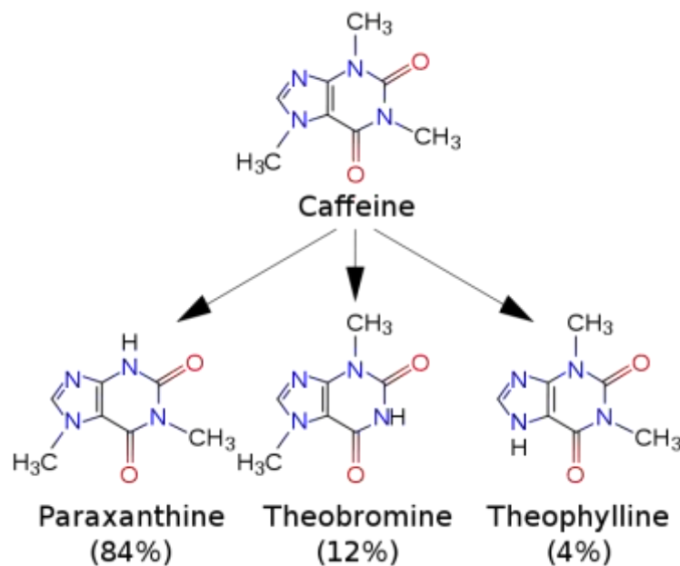
Figure 28 : métabolisation de la caféine en ses métabolites actifs (300).
