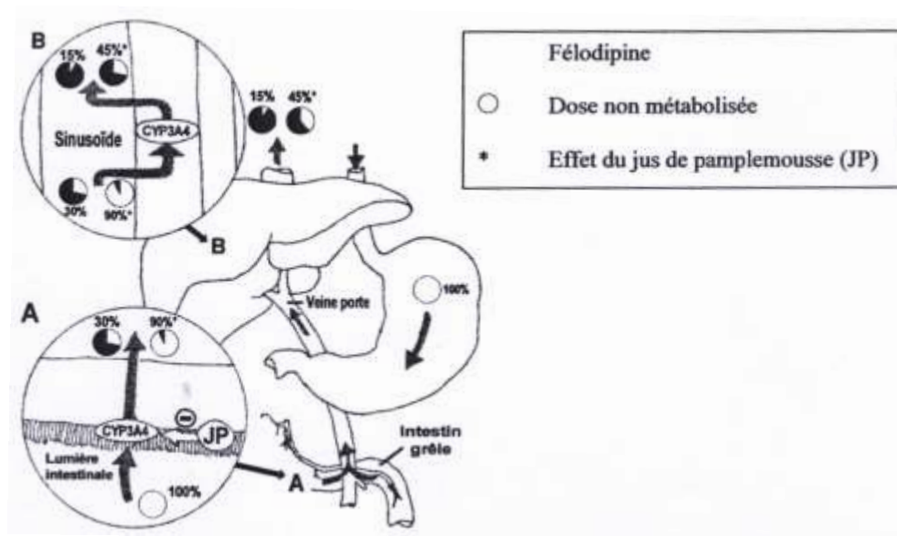
Figure 15 : métabolisme séquentiel présystémique de la féلودipine par le CYP 3A4 dans les entérocytes (A) et les hépatocytes (B) en absence et en présence de jus de pamplemousse (39).
