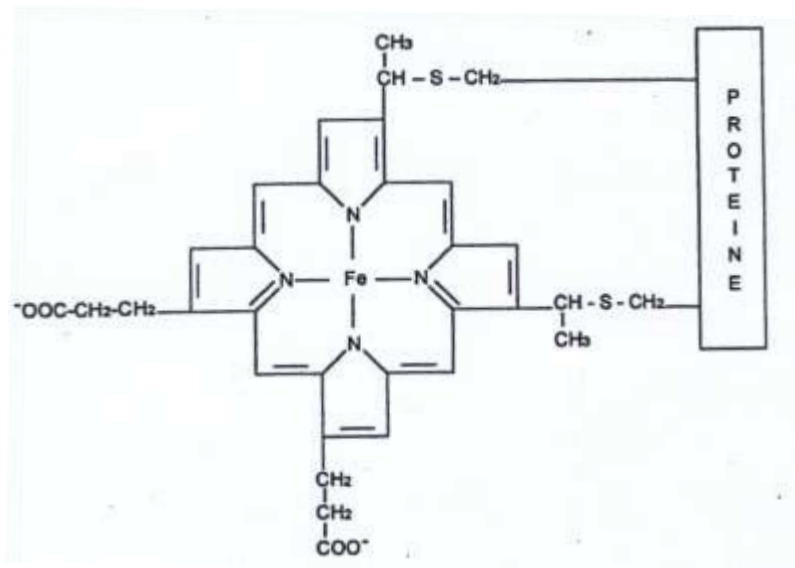
Figure 8 : structure d'un cytochrome P450 (11).
