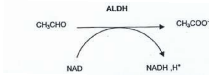
Figure 24 : oxydation de l'acétaldéhyde par l'ALDH
