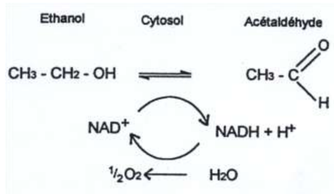
Figure 19 : réaction d'oxydation de l'éthanol par l'ADH (11).
