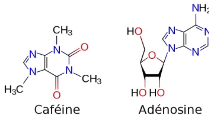
Figure 27 : molécules de caféine et d'adénosine (300).
