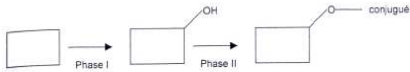
Figure 6 : résumé des deux phases d'une biotransformation d'un médicament.
