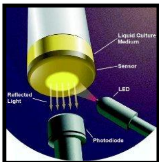
Figure 5 : Principe du faisceau de lecture.
