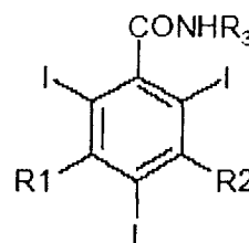
Structure d'un monomère non ionique
