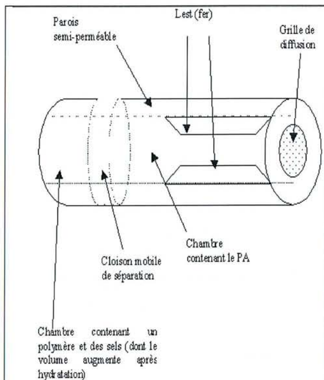
Figure 7 : Représentation schématique du bolus IVOMEC® (Laboratoire Merial) [42]
