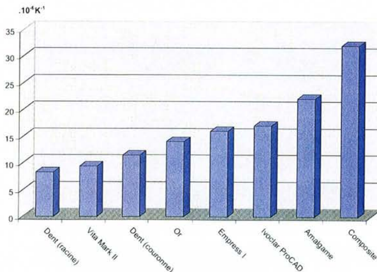
Coefficient de dilatation thermique de la dent et de certains matériaux de restauration courants [130]
