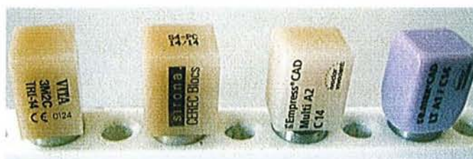
Blocs d'usinage en vitrocéramique et céramique feldspathique destinés au système Cerec®. On peut noter la couleur particulière du bloc IPS e.max CAD® qui après usinage devra être densifié secondairement par cristallisation
