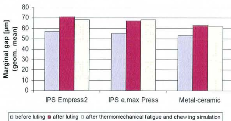
Gap marginal (en µm) sur des bridges 3 éléments Empress II®, e.max Press® et céramo-métallique avant et après collage, et après fatigue thermomécanique [183]
