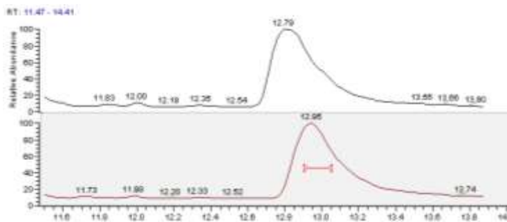
Figure 7 : Chromatogrammes du JWH018 lors des essais d'interférences. (a) urine surchargée en JWH018 ; (b) urine surchargée en JWH018 et en opiacés, cocaïne, cannabis et benzodiazépines ; (c) urine surchargée en JWH018, en amphétamines, en méthadone et buprénorphine.
