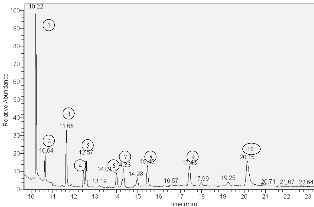
Figure 6 : Chromatogramme d'une urine surchargée à 100 ng/mL de cannabinoïdes de synthèse en mode TIC (Total Ionique Courant). 1: JWH250 ; 2 : RCS-4 ; 3 : JWH073 ; 4 : JWH018-D11 ; 5 : JWH018 ; 6 : AM2201 ; 7 : JWH122 ; 8 : JWH073-4-N-(hydroxybutyl) ; 9 : JWH018-5-N-(hydroxypentyl) ; 10 : JWH200.
