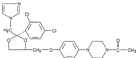
Ketoconazole
