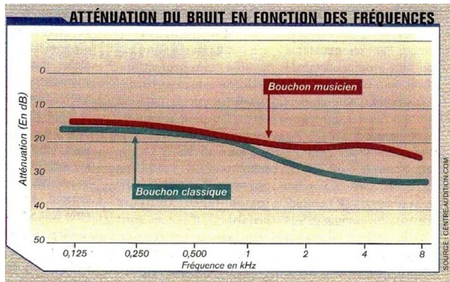
FIGURE 38 : ATTÉNUATION DU BRUIT DANS LES BOUCHONS POUR MUSICIENS
