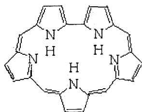
Sapphyrin
