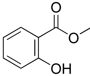
Figure 9 : Salicylate de méthyle
