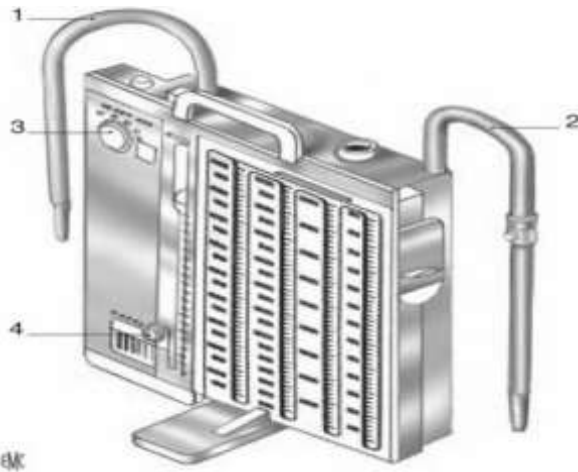
Fig 18. Système d'aspiration à usage unique. 1. Tuyau d'aspiration murale. 2. Tuyau relié au drain du patient. 3. Sélecteur de la force d'aspiration. 4. Visualisation du bullage et des oscillations.
