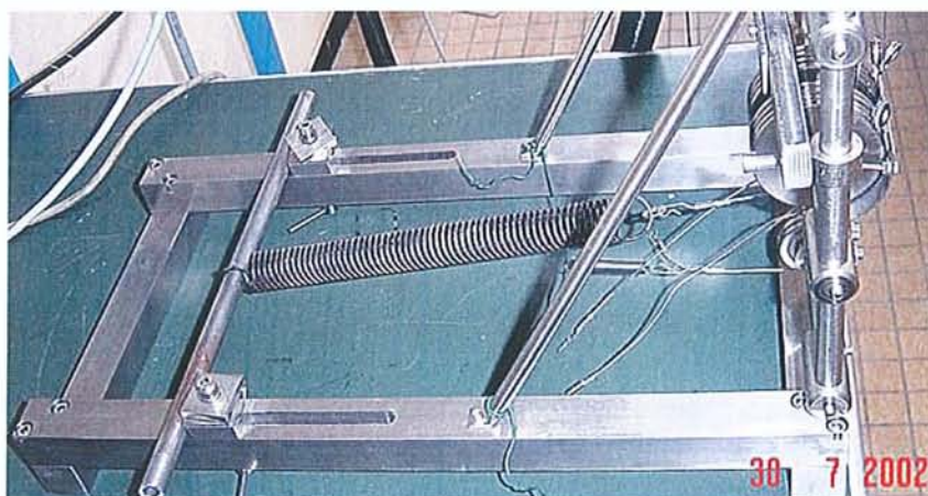
Étalonnage par traction sur un ressort préalablement taré.
