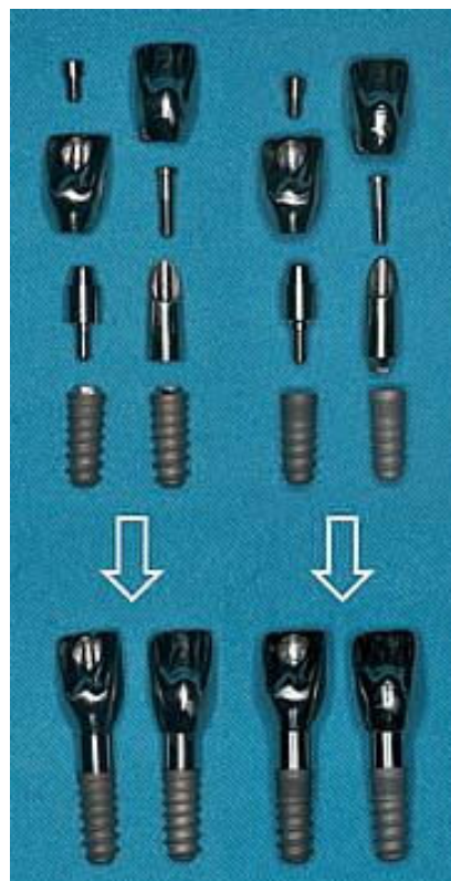
Illustration 20 : Prothèse vissée et scellée à connexion externe à gauche et à hexagone interne a droite. (Freitas AC Jr. et coll 2011).
