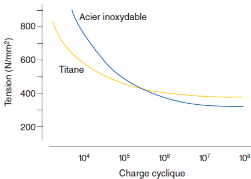
Illustration 73 : Résistance à la fatigue d'un implant en acier et en titane. (Altman M. et coll., 2012).
