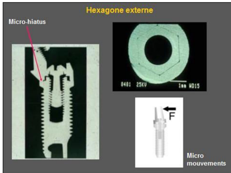
Illustration 38 : connexion externe adaptation (D'après Romanos GE., 2009).
