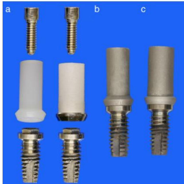
Illustration 81 : (a) pilier plastique calcinable. (b) pilier plastique calcinable avec bague usinée. (c) piliers une fois coulés. (Do Nascimento C. et coll., 2009).
