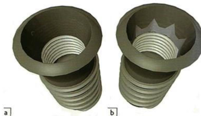
Illustration 19 : a) Connexion cône morse pur. b) cône morse indexé (d'après Szmukler-Moncler S. et coll, 2008).
