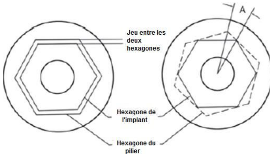
Illustration 79 : Représentation du jeu en rotation (Kano SC. Et coll., 2007).
