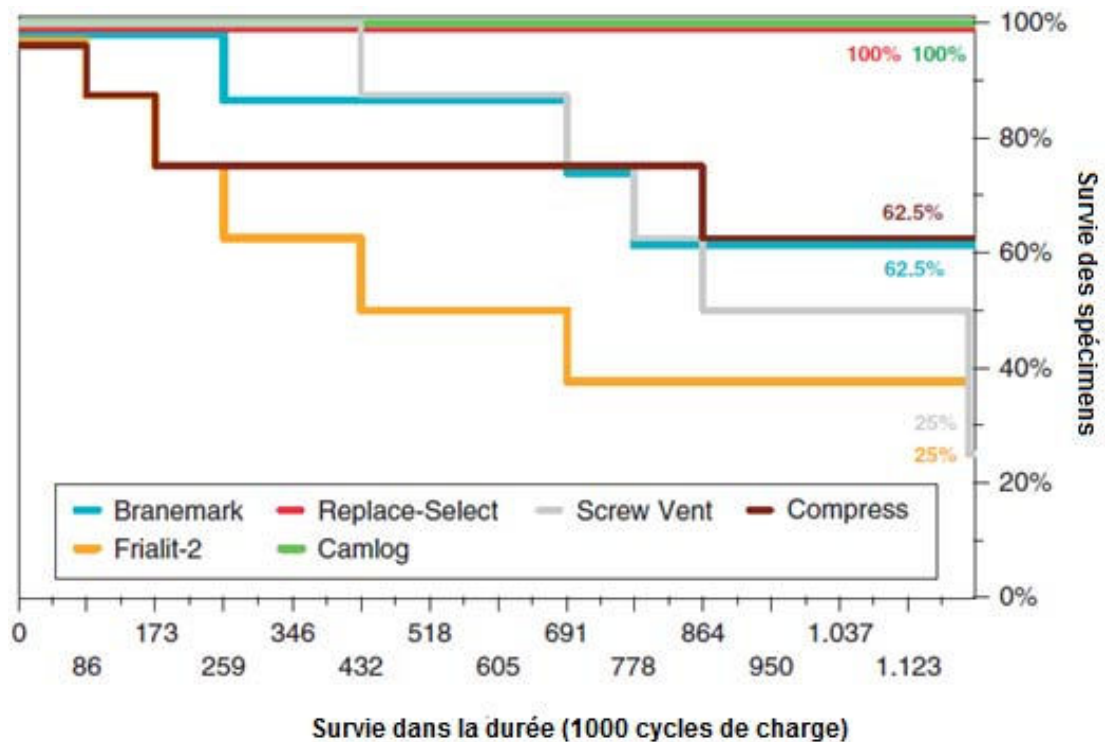
Illustration 75 : Comparaison entre différentes connexions à épaulement horizontal. (D'après Steinebrunner L. et coll., 2008).
