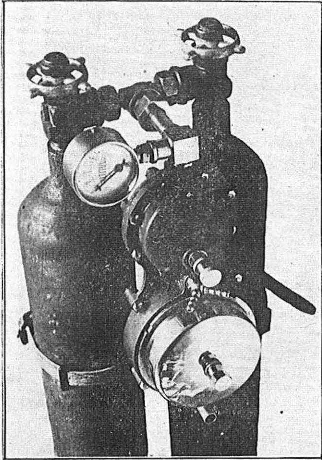
Fig. 2. — Détendeur monté sur deux réservoirs à gaz jumelés
