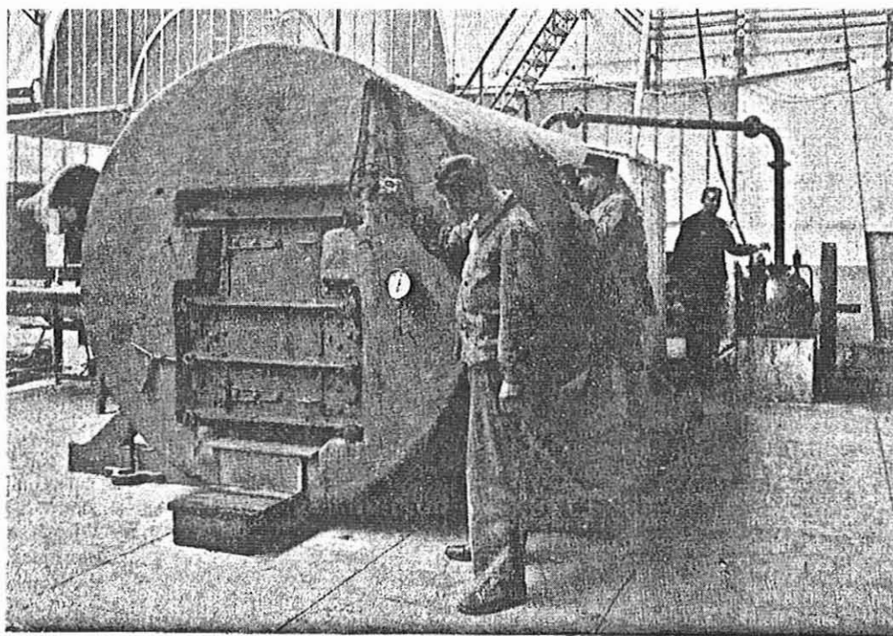
Fig. 1. — La caisse pneumatique de l'Institut aérotechnique de Saint-Cyr pendant une expérience. Le physiologiste observe le sujet enfermé dans la chambre grâce à un hublot. L'aide régle les soupapes par le volant à main et le mécanicien surveille la pompe.
