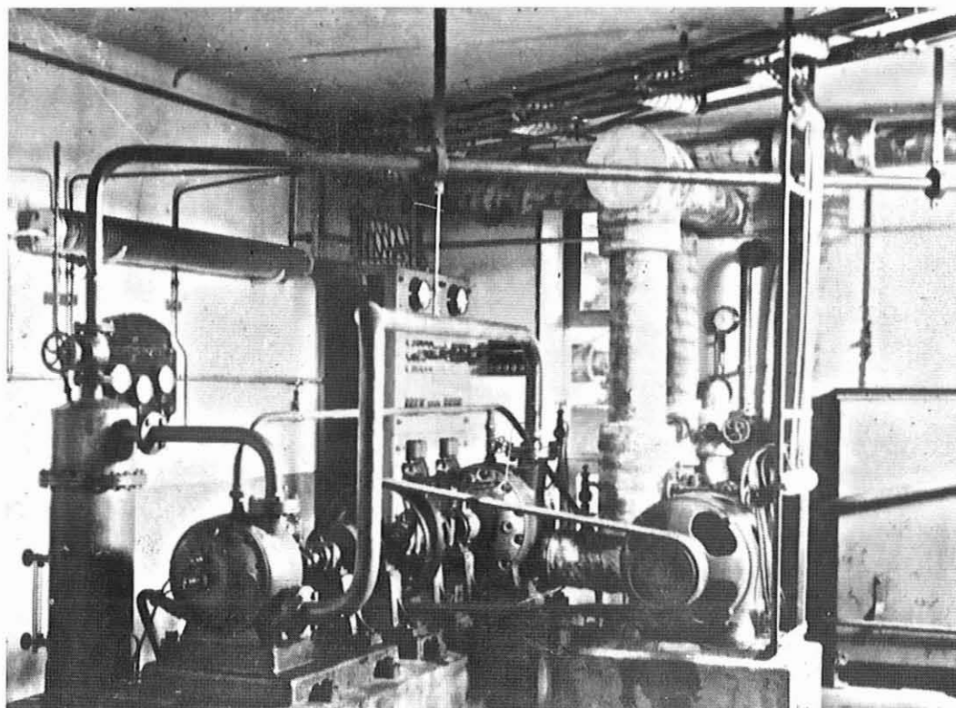
Image 45 : la machinerie à dépression et à froid Histoire Anecdotique de la Médecine de l'Air. 1963. Docteur GARSAX. Exemplaire sous presse du Centre de Documentation du Musée de l'Air et de l'Espace
