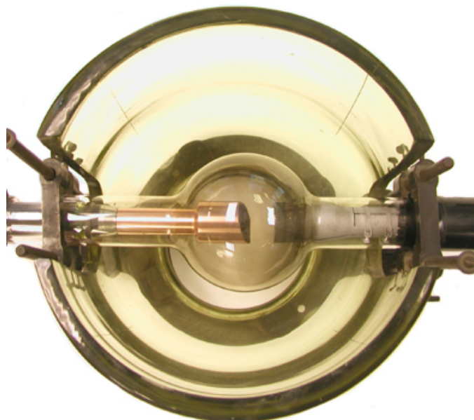
Figure 96 : La cupule protectrice en verre plombé (Health Physics, 2012)
