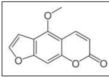
Figure 22 : Bergaptène
