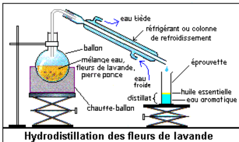
Figure 5 : Schéma d'une hydrodistillation (Source : Couic-Marinier F. et Lobstein A., Les huiles essentielles en pratique à l'officine)
