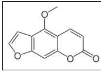
Figure 22 : Bergaptène
