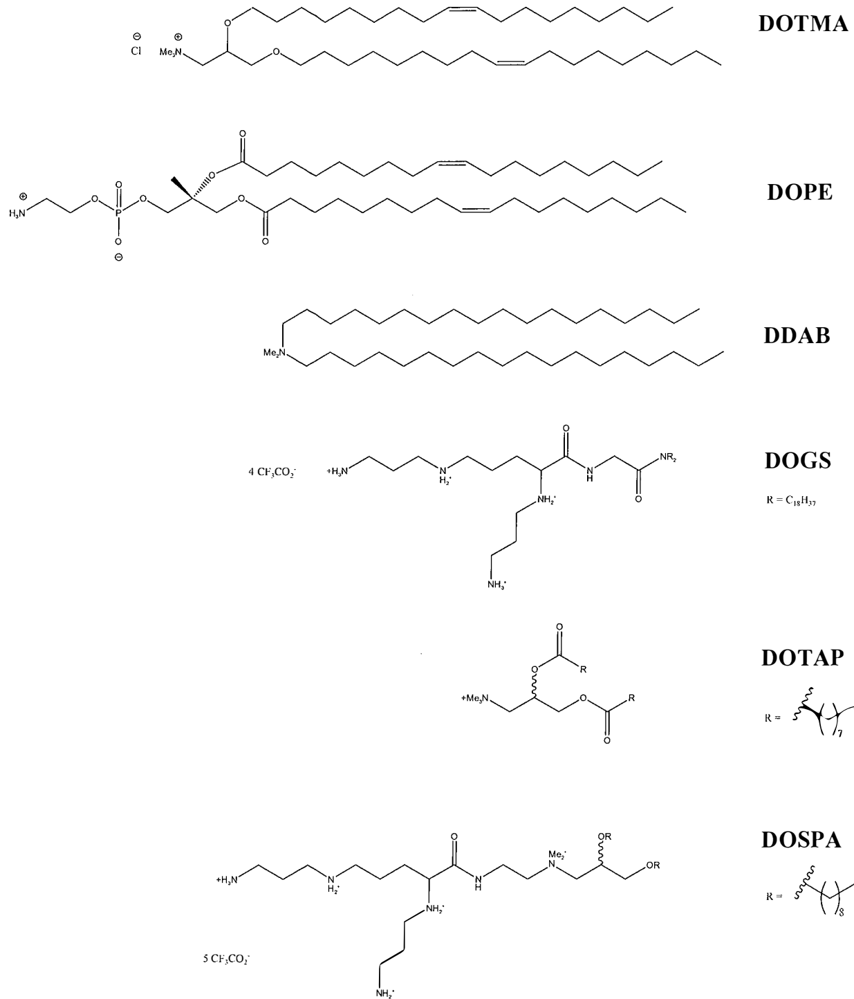
Schéma 11 : Principaux lipides cationiques
