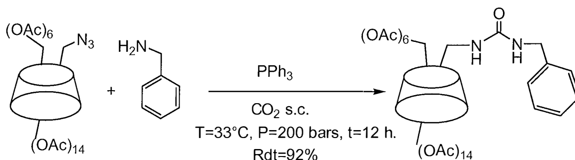
Schéma 23 : La réaction phosphinimide en \text{CO}_2 supercritique R=92\%
