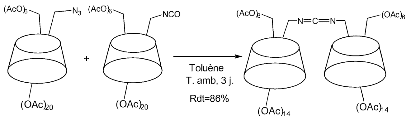
Schéma 25 : Synthèse du carbodiimide
