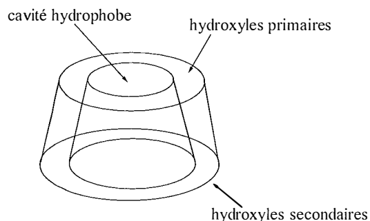
Figure 2 : aspect tridimensionnel d'une cyclodextrine
