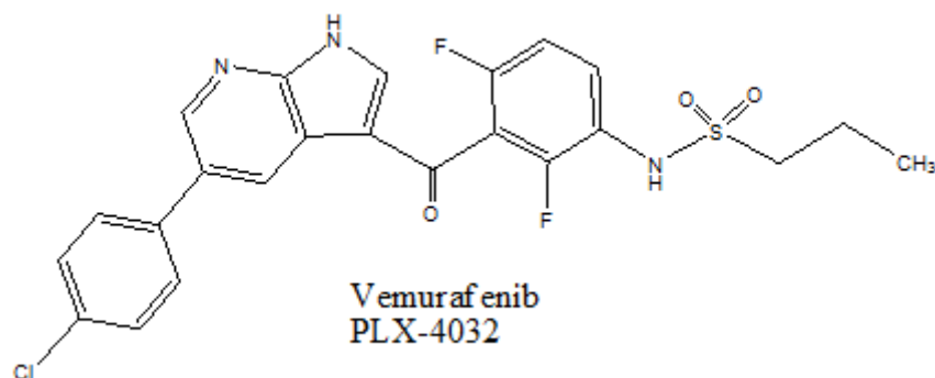
Figure 28 : Formule chimique du vémurafénib
