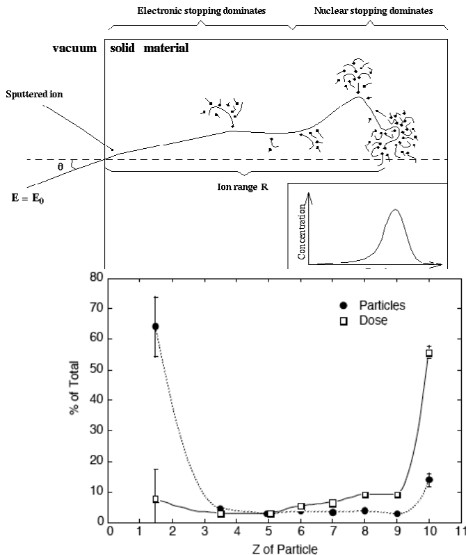
Figure 11 : Spectre de fragmentation des ions néon (Z=10) traversant 16 cm d'eau et dose relative déposée par chaque fragment.
