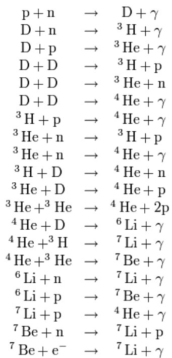
Figure 103 : réactions de la nucléosynthèse primordiale
