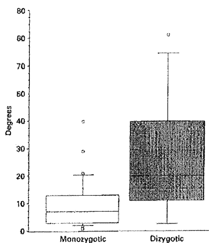
Fig.11 – Différence significative de sévérité des courbures entre des jumeaux monozygotes et des dizyotes (95). Les traits horizontaux représentent les 10 ème et 90 ème percentiles et les rectangles les 25 ème , 50 ème et 75 ème percentiles. Les cercles indiquent les individus au-delà du 10 ème percentile dans chaque direction
