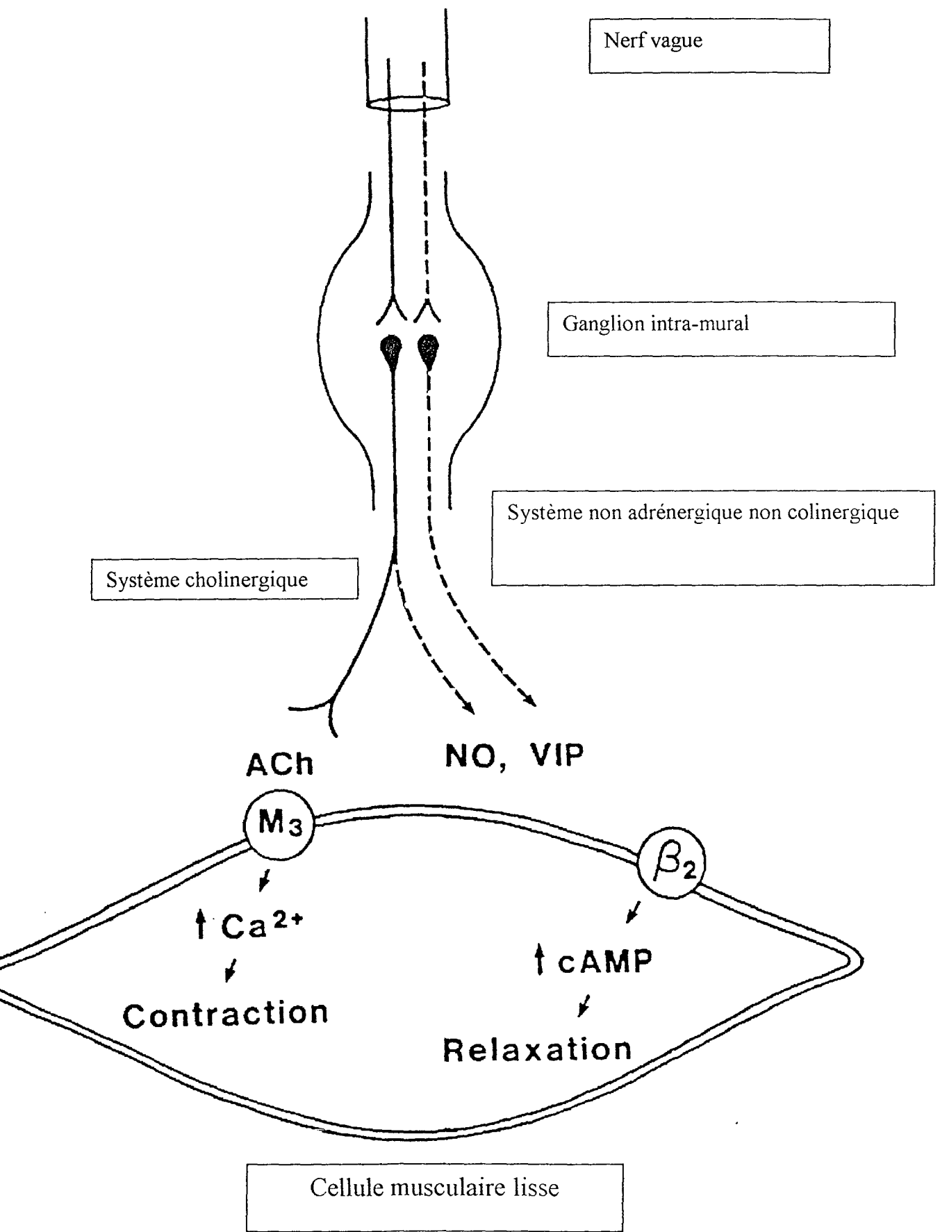
Schéma 2: innervation cholinergique et système non adrénérique non cholinergique
