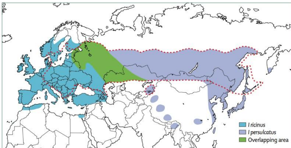
Figure 3: Répartition géographique d' Ixodes ricinus et d' Ixodes persulcatus [16]
