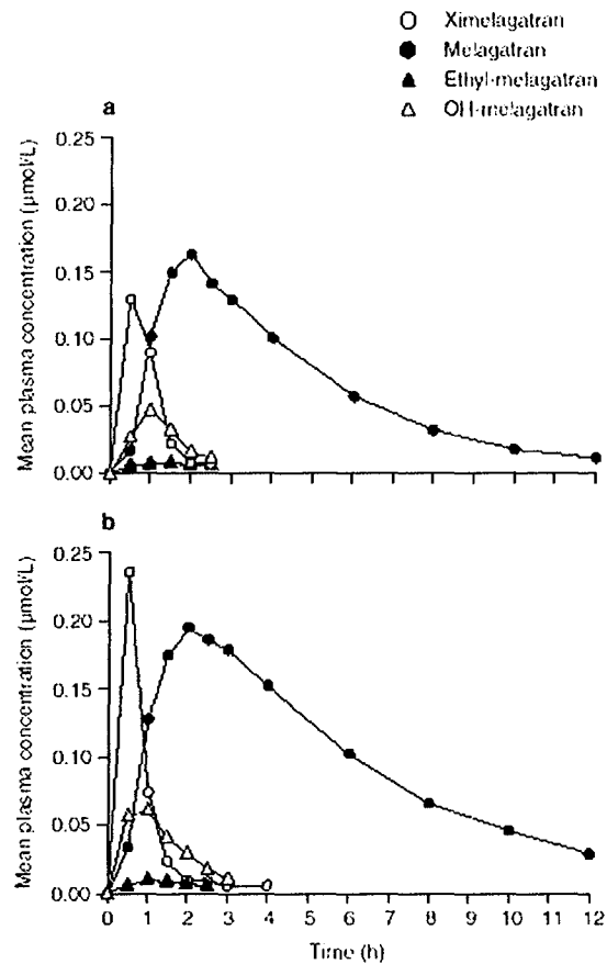
Figure 36: Evolution de la concentration plasmatique de ximélagatran, mélagatran, ethylmélagatran et mélagatran hydroxyamidine en fonction du temps après administration par voie orale de 20 mg de ximélagatran à des sujets sains jeunes (a) ou âgés (b)
