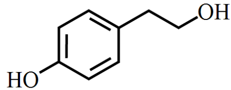
Figure 22 : Structure du p-tyrosol (25)
