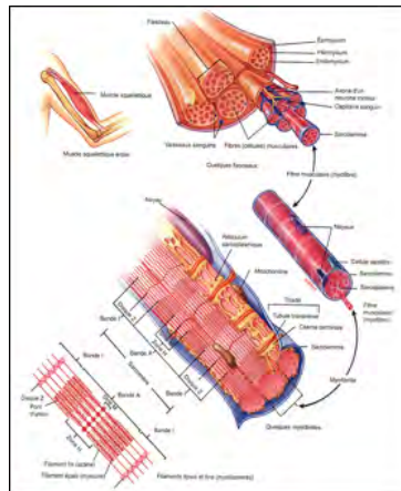
FIGURE 2.3: Anatomie du muscle strié squelettique
