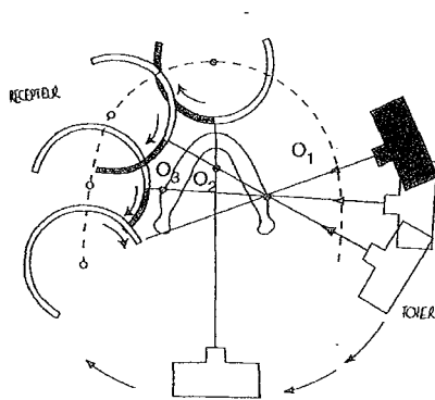
Principe de la radiographie panoramique
