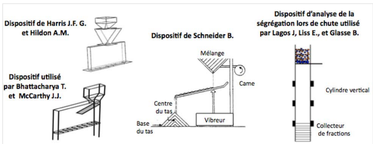
Figure 33 : Exemple de dispositifs d'analyse de la ségrégation lors de la chute [MASSOL-CHAUDEUR, BERTHIAUX ET DODDS, 2003] [BHATTACHARYA et McCARTHY, 2014] [LAGOS, LISS et GLASS, 1999]
