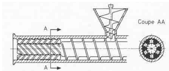
Figure 18 : Extrudeuse à satellites planétaires [BARBARIT, 1987, p. 18]
