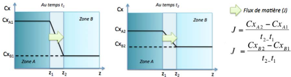
Figure 56 : Représentation du phénomène de diffusion [GERL, 1976]
