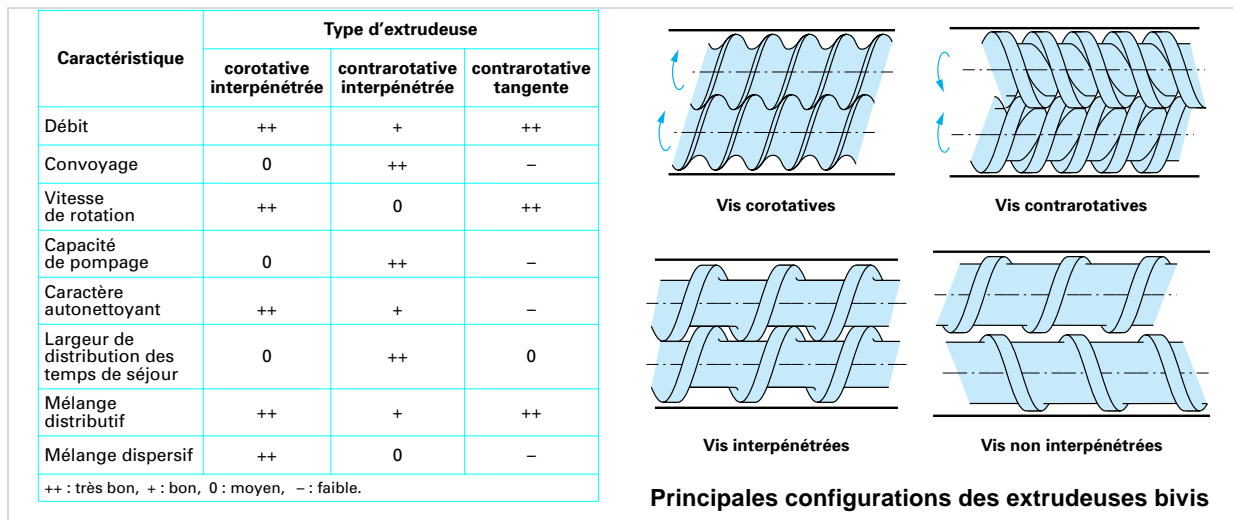
Figure 16 : Principales configurations des extrudeuses bivis : Caractéristiques et schémas [VERGNES et CHAPET, 2001].
