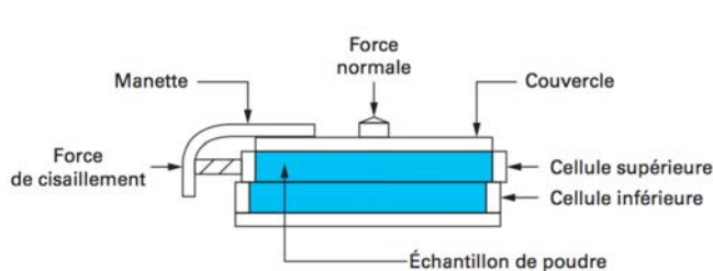
Figure 41 : Cellule de Jenike et essai de cisaillement [SALEH et GUIGON, 2012] [SCHER, 2006]
