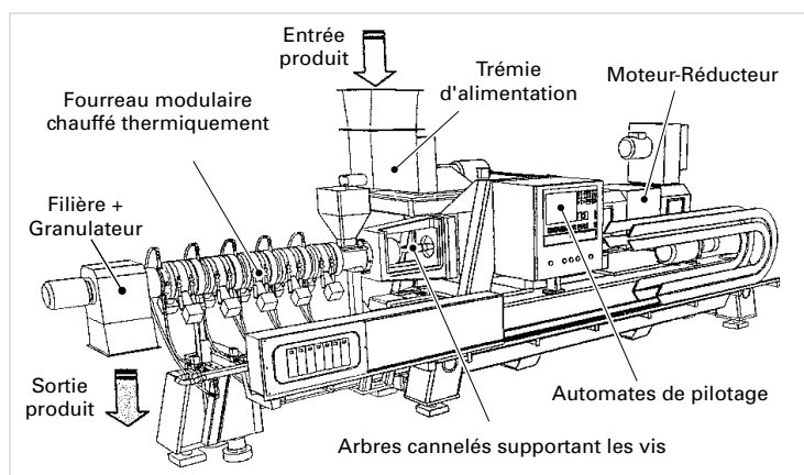
Figure 14 : Extrudeuse bivis (modèle Evolum 53, Clextral, 1999) [ROUSTEL, CHAPET et BOUVIER, 2000].
