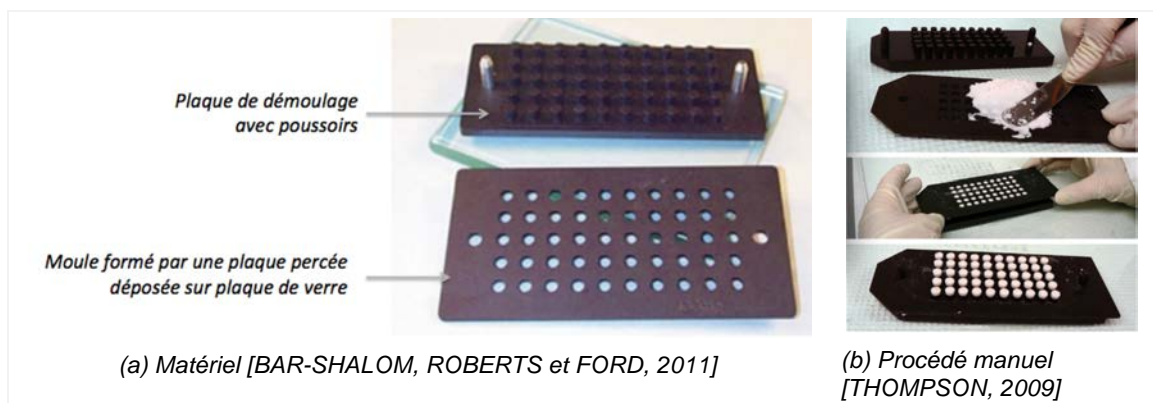
Figure 12 : Fabrication manuelle de comprimés par moulage. (a) matériel [BAR-SHALOM, ROBERTS et FORD, 2011] ; (b) mode opératoire [THOMPSON, 2009]
