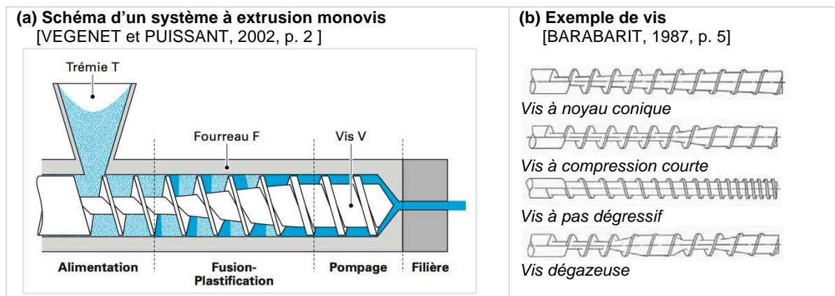
Figure 15 : Extrudeuse monovis [VEGENET et PUISSANT, 2001] [BARBARIT, 1987, p. 5]
