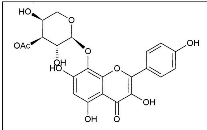
Figure n°35 : Structure de l'acétylrhodalgine [17]
