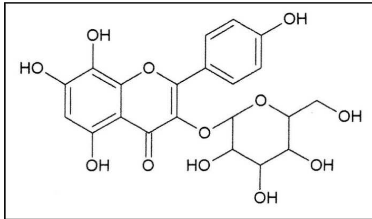
Figure n°31 : Structure de la rhodaline [17]
