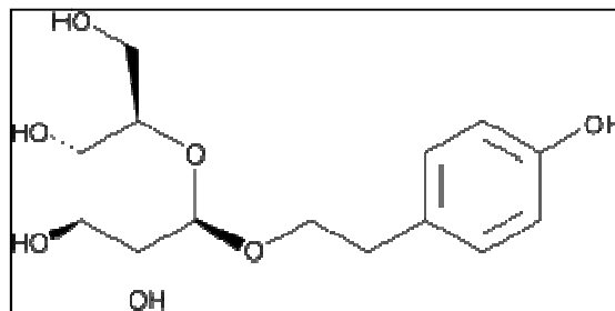
Figure n° 39: Structure du salidoside [17]
