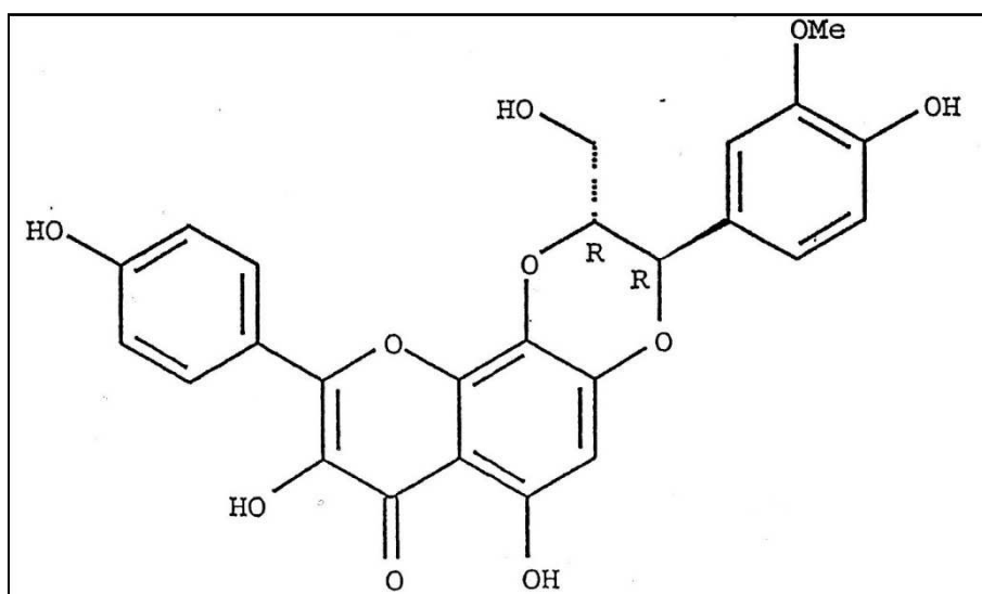
Figure n°30 : Structure de la rhiodoline [17]
