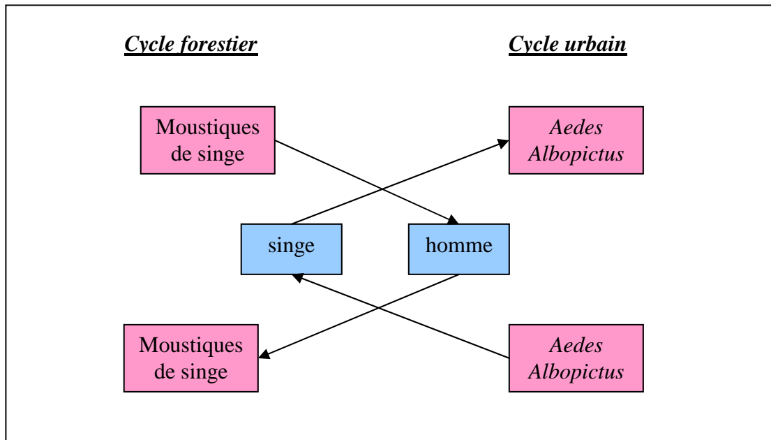
Figure n° 7 : Les 2 cycles du virus du Chikungunya : CHIKV (Huraux J.-M. et al. , 2003)
