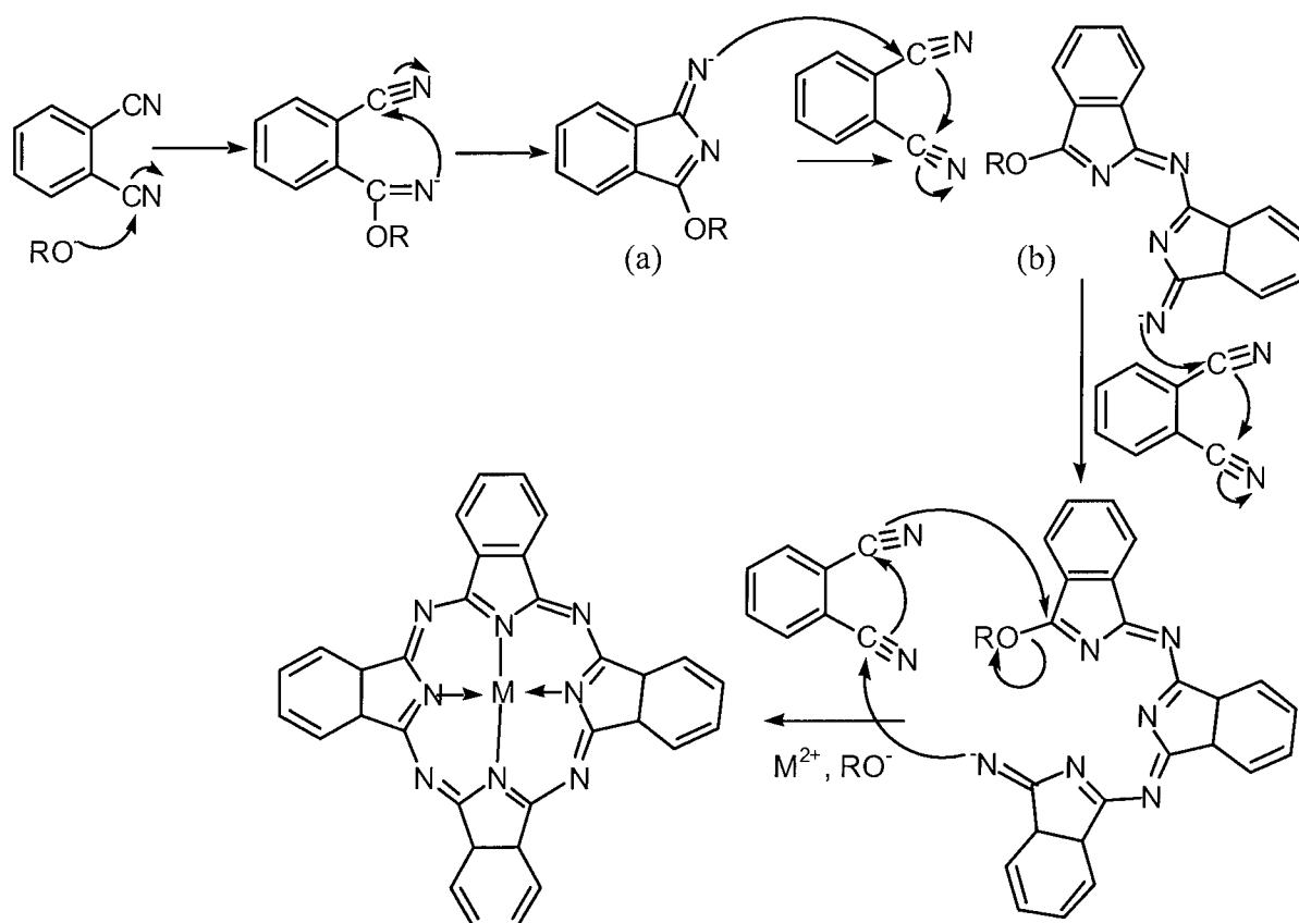
Figure 2 : cyclisation des phthalonitriles en phthalocyanine [9]
