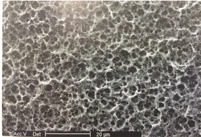
Figure 26: Vue au microscope électronique de l'état de surface microrugueux du zircon. (Gahlert, 2014)
