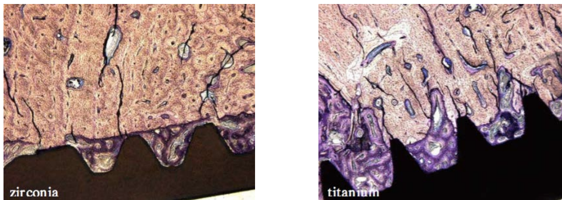
Figure 36: Coupe histologique de l'ostéo-intégration des implants en zirconie (à gauche) et titane (à droite) à quatre semaines. (Depprich Rita H. Z.-P.-C., 2008)
