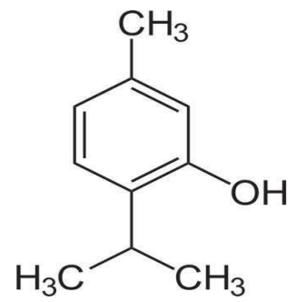
Figure 3 : le thymol
