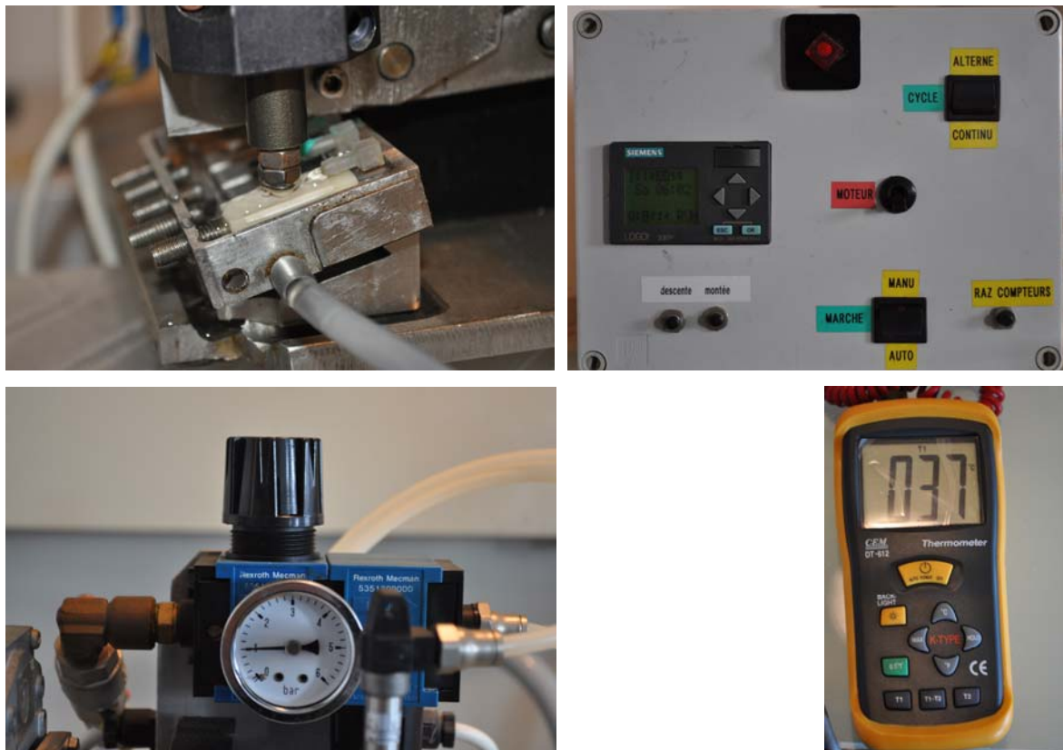
Fig 71. Vue en détail de l'indenteur, du programmateur, du manomètre et de la sonde de surveillance de température.
