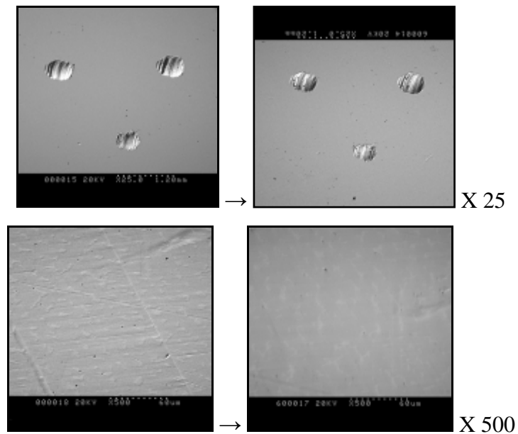
Fig 54. Vue au M.E.B. des échantillons de Cr-Co polis miroir avant et après le passage en solution.
