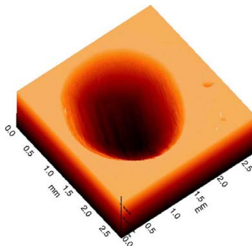
Fig 47. Exemple d'image obtenue par scannage 3D, d'après HEINTZE et Al. en 2006.
