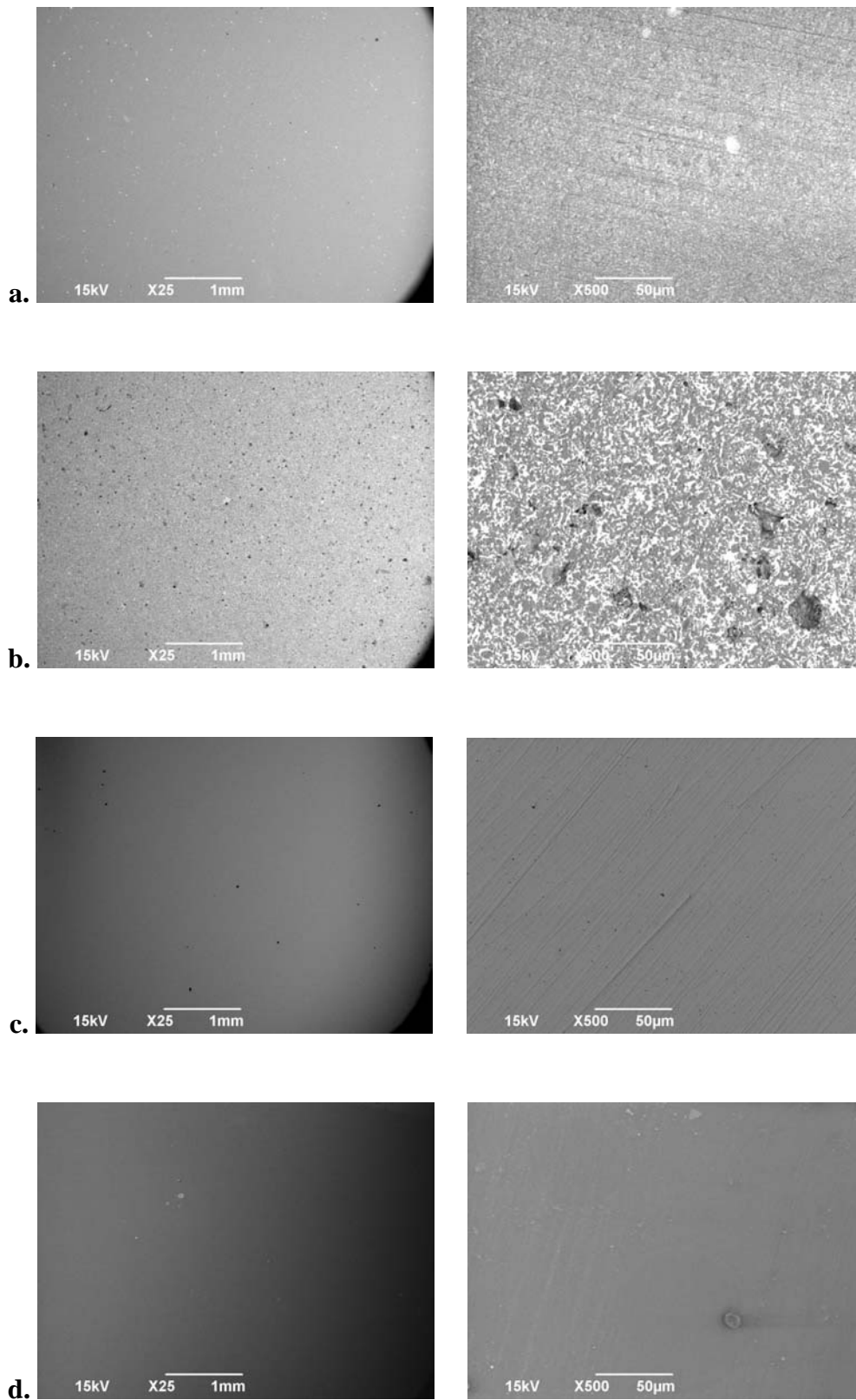
Fig 68. Vues au M.E.B. au grossissement 25X puis 500X des échantillons d'IPS e-max CAD (a.), d'In ceram Alumina (b.), de zircone (c.) et de résine (d.).
