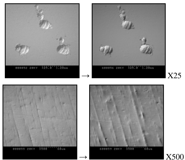
Fig 56. Vue au M.E.B. des échantillons de Ti-cp polis miroir avant et après le passage en solution.
