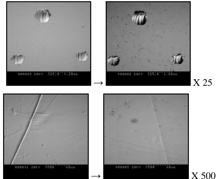
Fig 53. Vue au M.E.B. des échantillons d’Au-Pt polis miroir avant et après le passage en solution.
