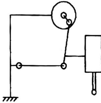
Fig 70. Schéma de la chaîne cinématique.
