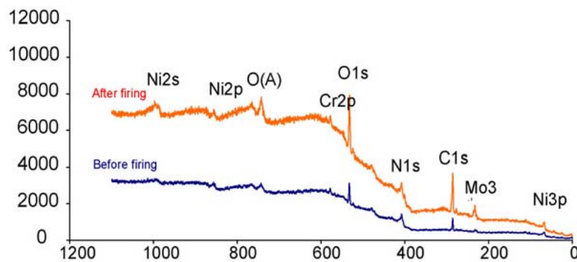
Fig 39. Exemple de courbe de résultat d'une XPS sur alliage de Ni-Cr avant et après cuisson de la céramique, selon [LIN, 2008].
