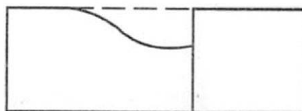
Fig 28. Schéma d'une corrosion par couplage galvanique entre un alliage noble, à droite et un alliage non noble, à gauche, selon [UPADHYAY, 2006].
