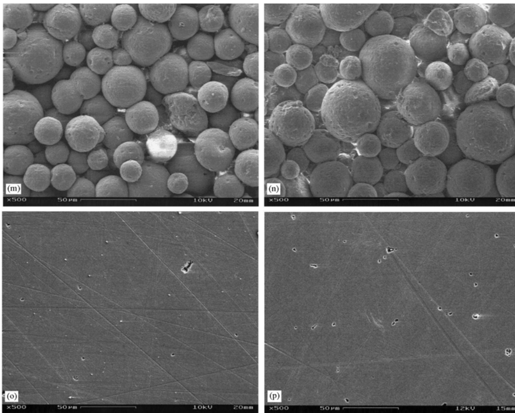
Fig 38. Exemple de vue de l'état de surface d'une céramique avant et après attaque, au MEB, selon [MILLEDING, 1999].
