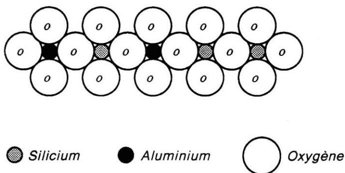
Fig 1. Structure des céramiques : représentation d'une chaîne aluminosilicique. D'après [OGOLNIK, 1992]
