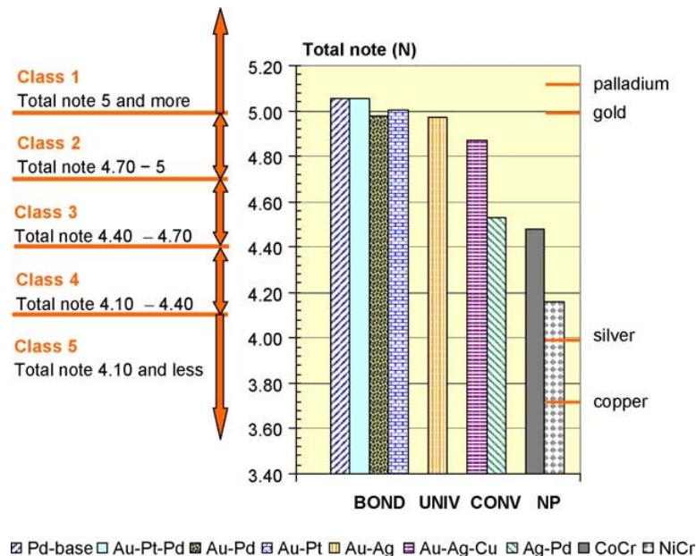
Fig 19. Corrosion des alliages dentaires, système de classification, selon [MANARANCHE, 2007].
