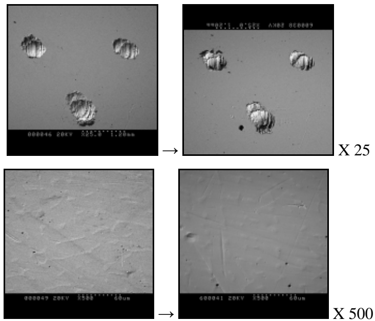
Fig 55. Vue au M.E.B. des échantillons de Ni-Cr polis miroir avant et après le passage en solution.
