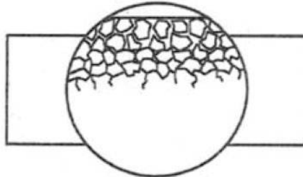
Fig 30. Schéma d'une corrosion intergranulaire, selon [UPADHYAY, 2006].
