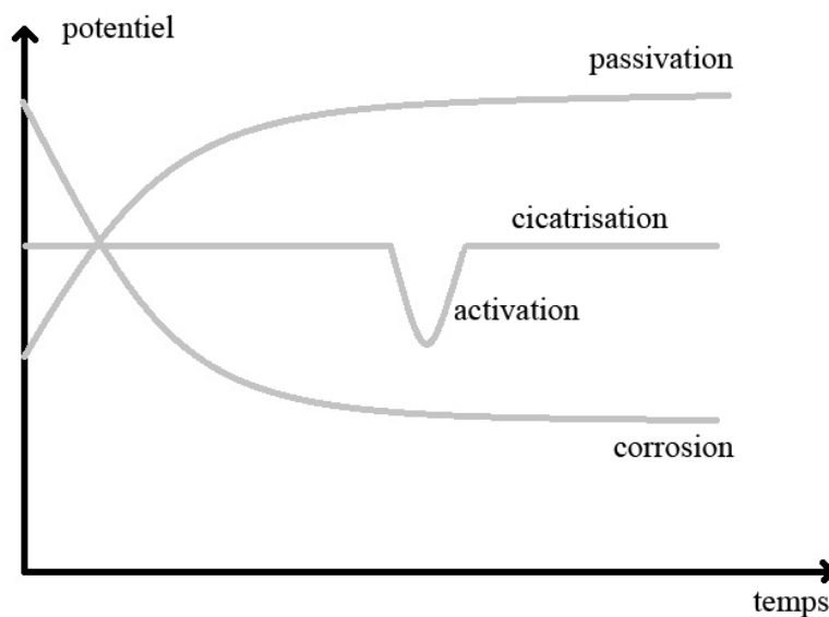
Fig 43. Courbes de potentiels de repos en fonction du temps. L'allure de la courbe correspond au comportement électrochimique.
