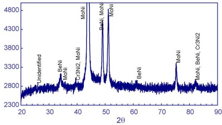
Fig 40. Exemple de courbe de résultat d'une XRD sur un alliage de Ni-Cr, selon [LIN, 2008].
