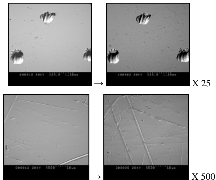
Fig 52. Vue au M.E.B. des échantillons d’Au-Pd polis miroir avant et après le passage en solution.
