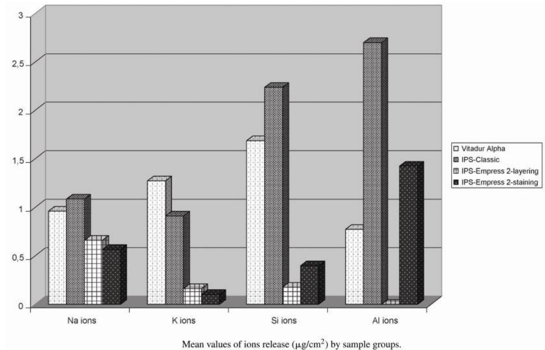
Fig 9. Principales valeurs de relargage ionique ( \mu\text{g}/\text{cm}^2 ) en fonction de l'échantillon, d'après [JAKOVAC, 2006].
