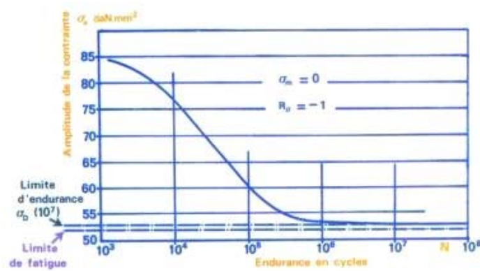
Fig 26. Variation de la contrainte maximum en fonction du nombre de cycle.
