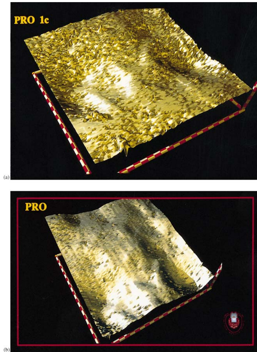
Fig 41. Exemple d'image obtenue par profilométrie laser, selon [MILLEDING, 1999].
