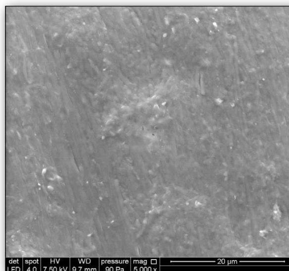
Figure 2 : surface amélaire, vue en microscopie électronique à balayage environnementale (grossissement X5000) (photo : S. Jager et E. Mortier)
