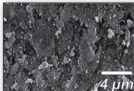
Figure 26 : micrographie d'une surface amélaire mordancée chimiquement et brossée (Hitmi et coll. , 2002)
