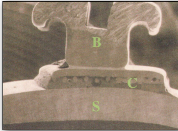
Figure 1 : coupe longitudinale d'un assemblage collé (bracket / colle / substrat). C : Colle, B : Brackets, S : Substrat (Hitmi et coll., 2002)
