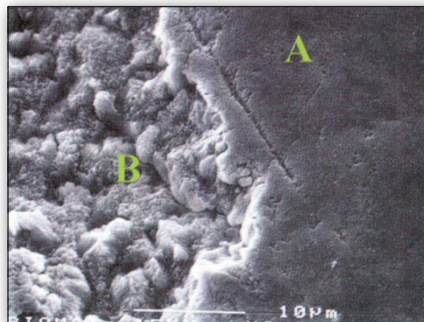
Figure 5 : micrographie d'une surface amélaire au microscope électronique à balayage. En A, la surface n'a subi aucun mordantage acide. En B, la surface a subi un mordantage à l'acide phosphorique (37 % pendant 30s) (x 2700) (Hitmi et coll., 2002)
