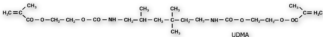
Figure 13 : représentation schématique de la molécule d'UDMA (Van Meerbeek et coll., 2003)
