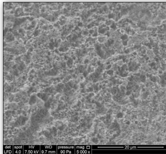
Figure 4 : surface amélaire (même dent et même zone que la figure 2) après mordantage à l'acide orthophosphorique à 34,5 % pendant 30 secondes, vue en microscopie électronique à balayage environnementale (grossissement X5000) (photo : S. Jager et E. Mortier)
