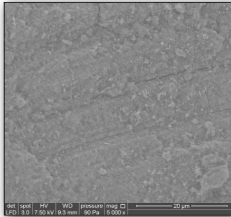
Figure 18 : surface dentinaire sans traitement de surface préalable, les tubulis ne sont pas décelables car recouverts par les boues de fraisage, vue en microscopie électronique à balayage environnementale (grossissement X5000) (Mortier et coll., 2011)
