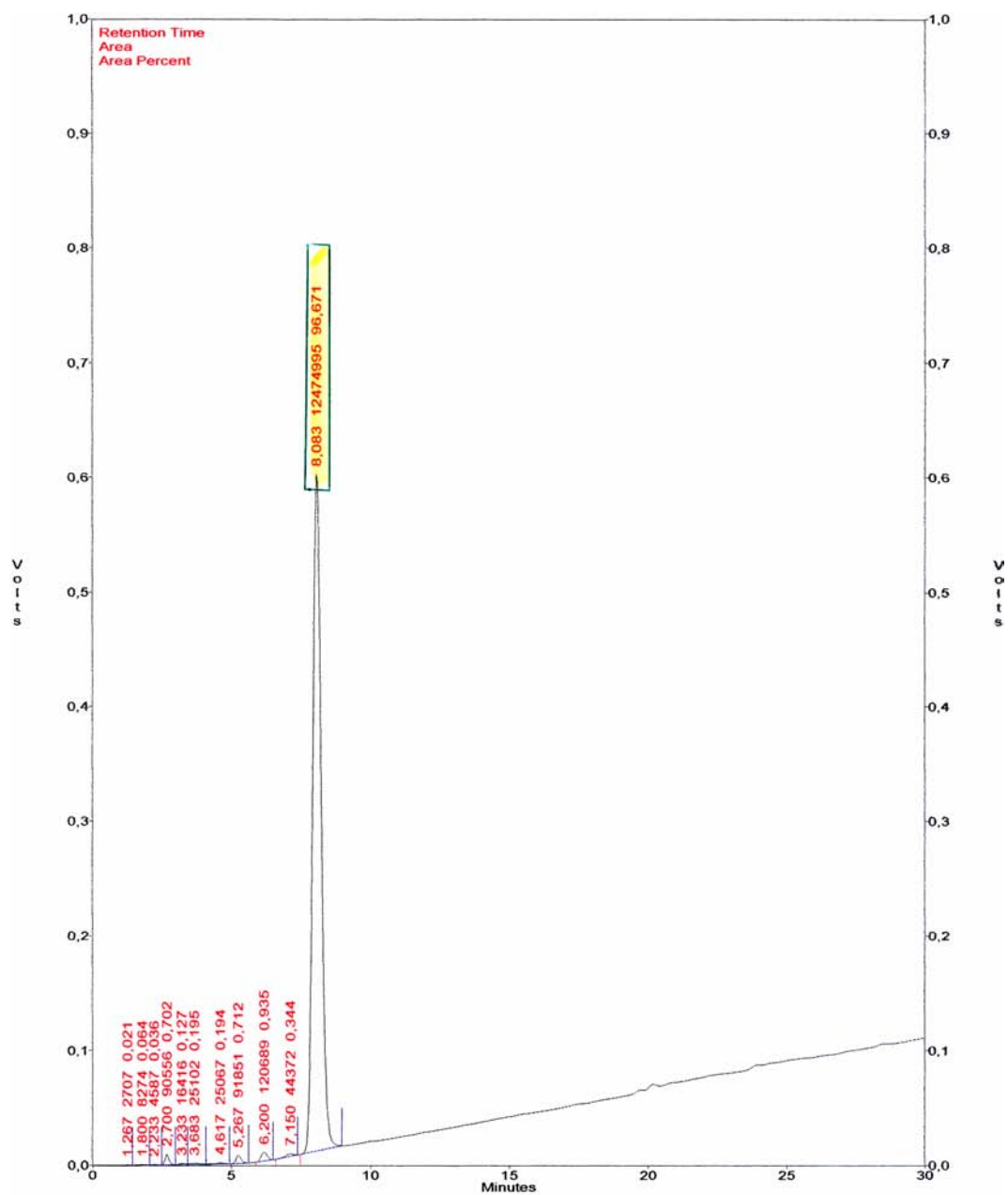
FIGURE 4.3 – Échantillon étalon de 10-décétylbaccatine III
