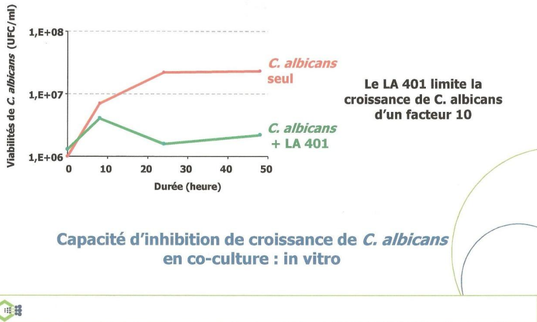
Figure 24 : Effet du L.acidophilus LA 401 sur le Candida albicans (Document IEDM).
