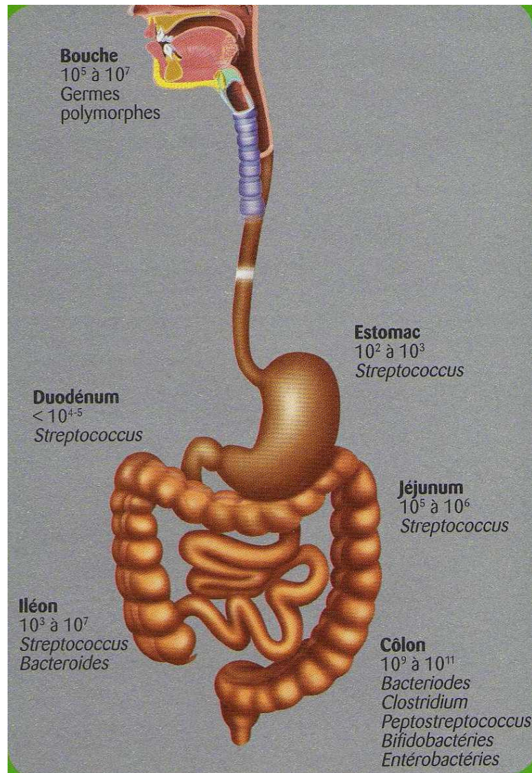
Figure 9 : Microbiote intestinal au fil du tractus digestif. (Mouton, 2007)
