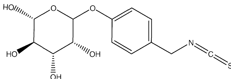
4(L-rhamnopyranosyloxy)benzylisothiocyanate 4RBITC
