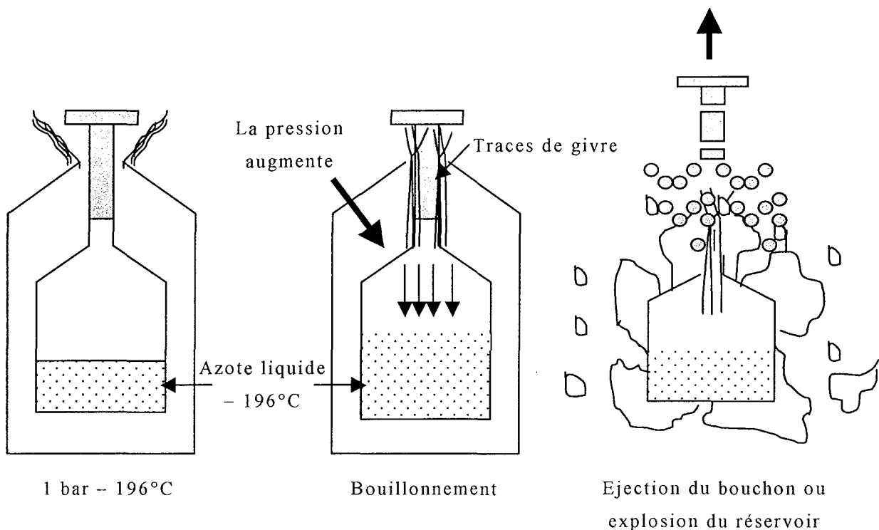
Figure 9 : le risque de surpression de l'azote liquide - 196°C
