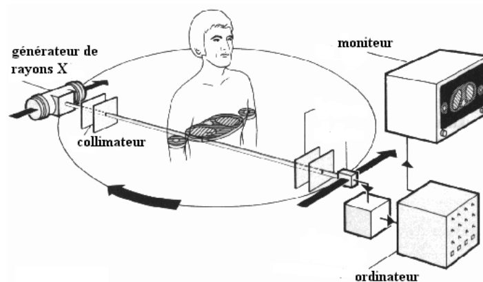
Figure 24 : Principe du scanner
