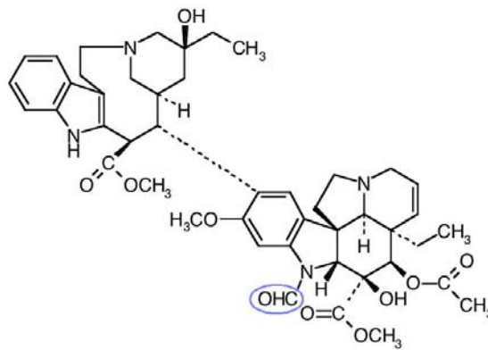
Figure 37 : Structure chimique de la Vincristine.
