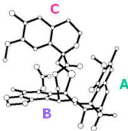
Figure 60 : Structure tridimensionnelle de l'ET- 743.
