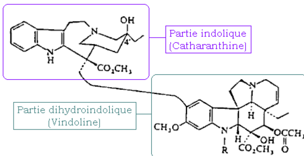
Figure 34 : Structure de base des Vinca-alcaloïdes.
