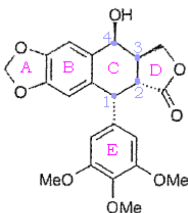
Figure 50 : Structure de la Podophyllotoxine, base de la synthèse de l'Etoposide et du Ténoposide.
